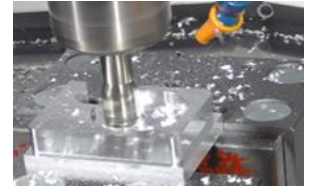
マシニングセンタによる切削加工
