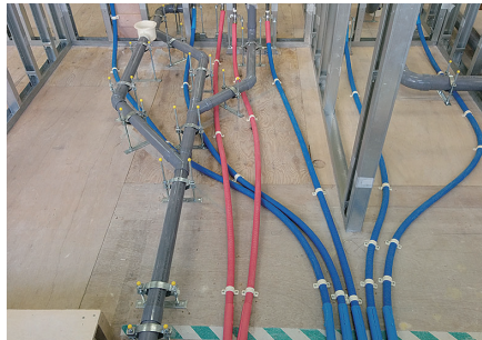
写真⑧：建築設備（配管の施工）
